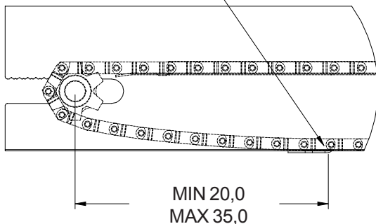
DÉTAIL DE LA TENSION DE LA CHAÎNE
